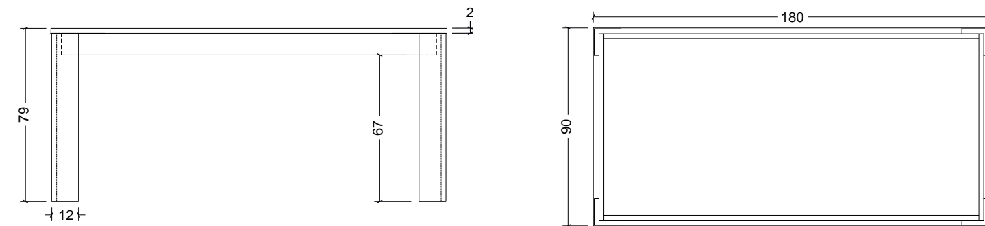
MESA DE COMEDOR 180x90 cm
